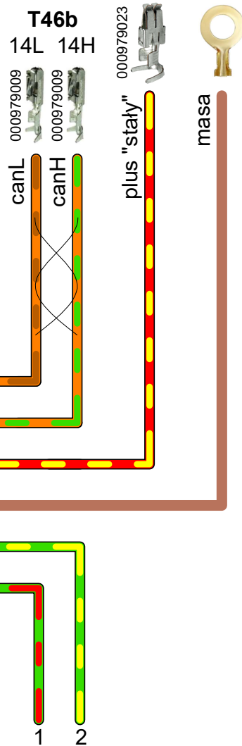
Złącza - przód, prawa strona
